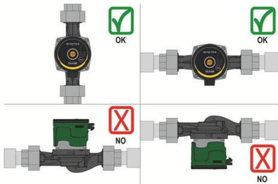
Рисунок 3: Монтажное положение
