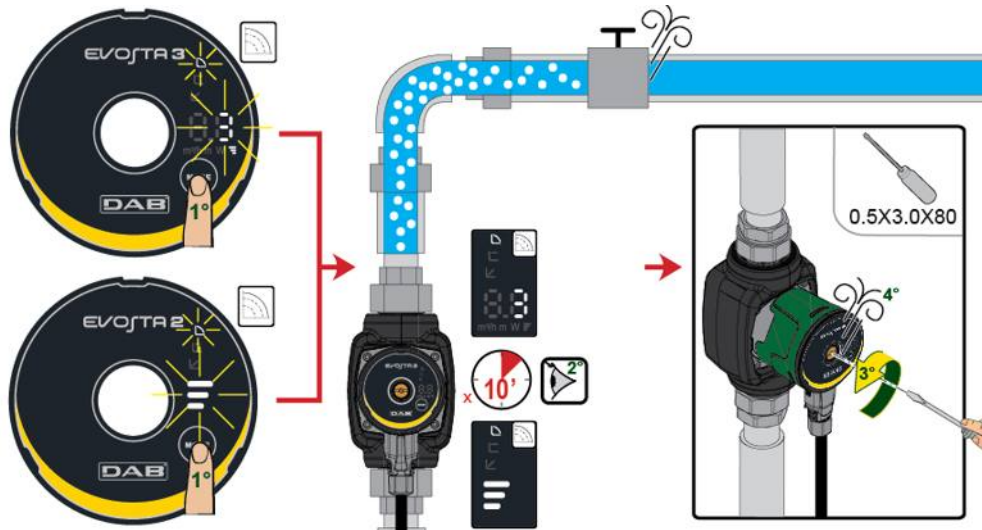
Obrázok 8: Odvzdušnenie čerpadla
