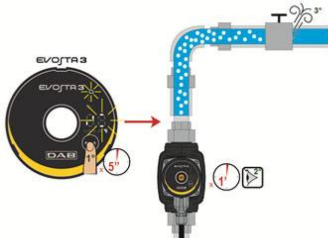
Abb. 9: Automatische Pumpenentlüftung
