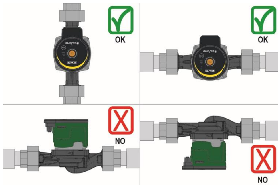
Εικόνα 13: Θέση συναρμολόγησης
